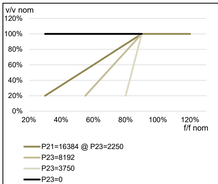
fig. 11B: Spannungssteigung im Unterdrehzahlschutz, P[23]
