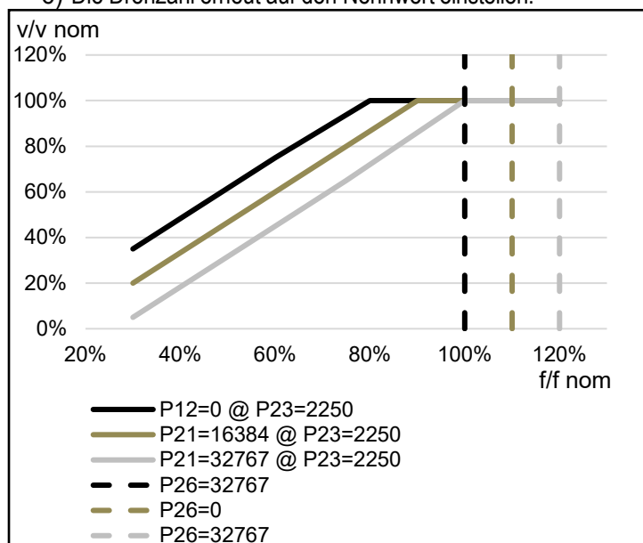
fig. 11A: Unter- und Überdrehzahlschutz, P[21] e P[26]
