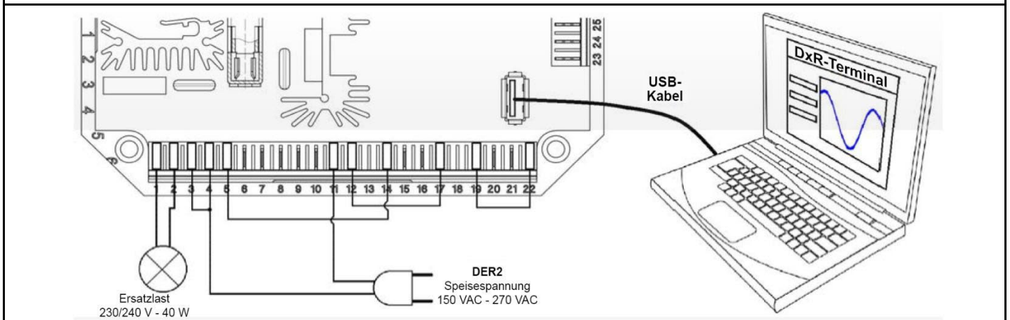
Abb. 13c: 150-270 VAC-Stromversorgung des DER2 für die Prüfung und Einstellung. (Bitte beachten Sie die Lastnachbildung zwischen den Klemmen 1 und 2, die Erfassung an Klemme 4 und die Brücken zwischen den Klemmen 5 und 14, 12 und 17, 19 und 22)
