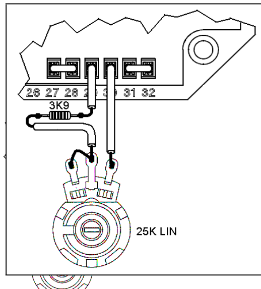
Abb. 5b: Anschluss des externen Potentiometers mit 25K
